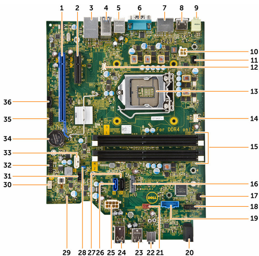
1. ábra. Az alaplap alkatrészei
